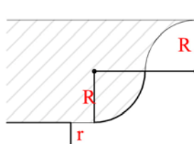
Figure 4-28 : Doucine droite
