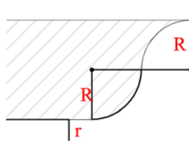
Figure 0-6 : Doucine droite
