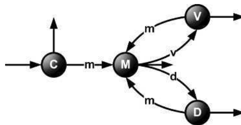
Figure 5.33 Cet automate est déterministe.
