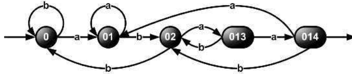
Figure 5.5 Automate déterminisé
