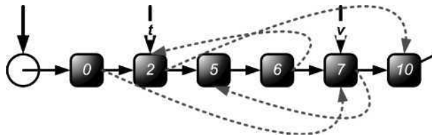
Figure 2.8 Permutation : le cas général...
