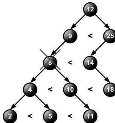
Figure 4.16 On veut supprimer le 8
