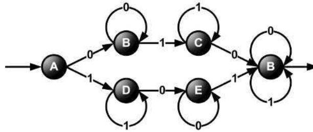
Figure 5.37 Cet automate est déterministe.
